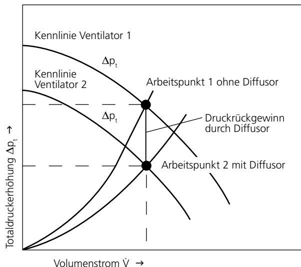
Bild 2: Druckrückgewinnung
