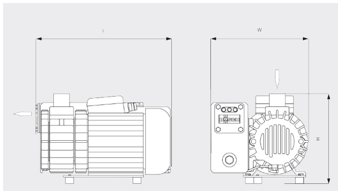
Rozměrový výkres
