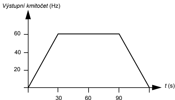
30sekundová křivka rampy zrychlení a zpomalení
